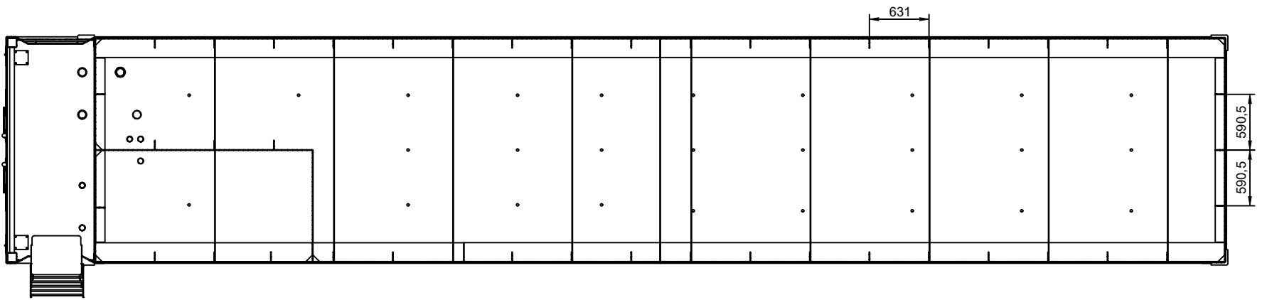
Section A-A Scale 1:40
